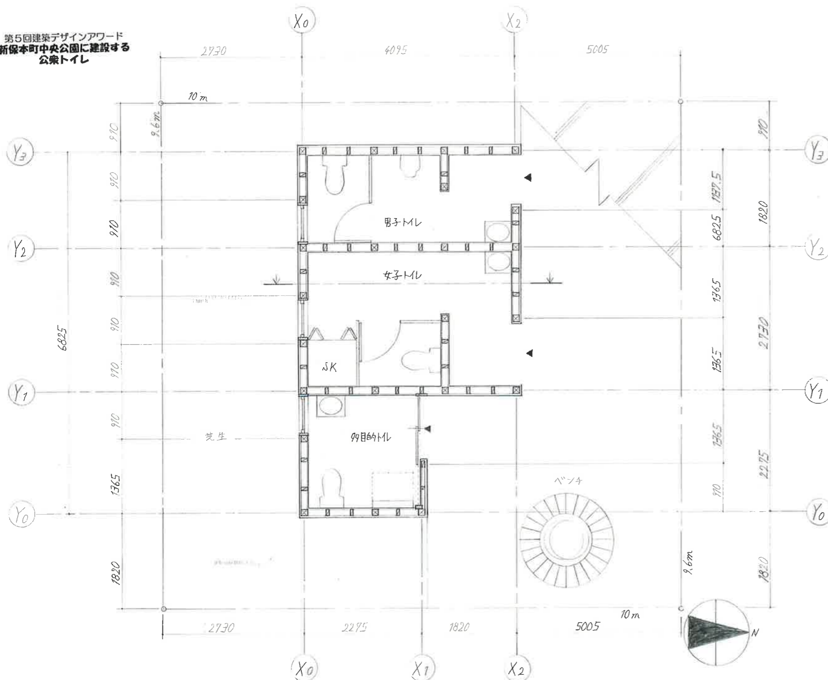
配置兼平面図 1:50
